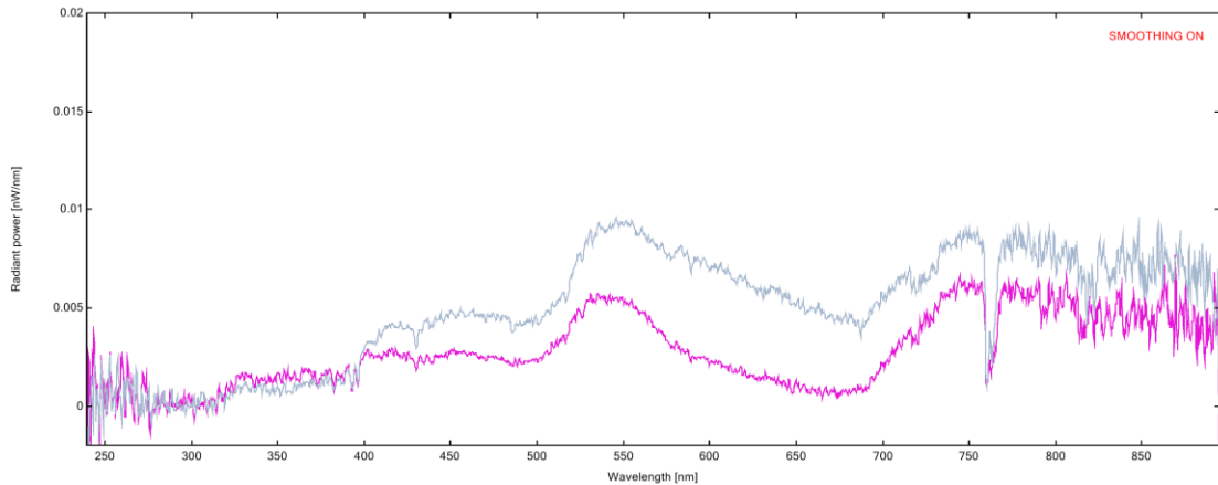
Nitrogénhiányos (kék) és kontroll növény reflektancia-spektruma
